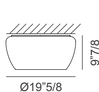
Implode PL 50
