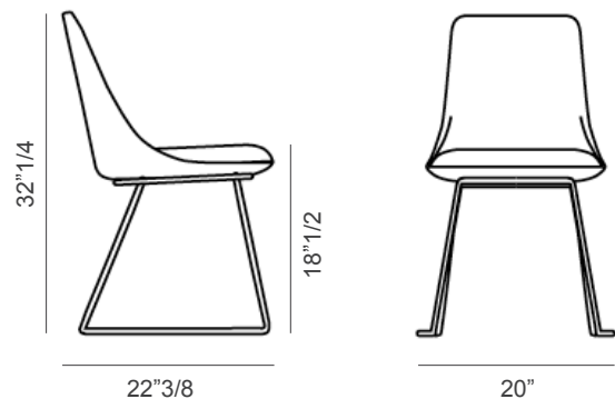
Sled base
