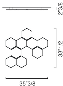
(D) 7370/A
