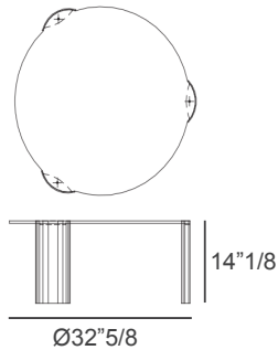
Round - B)
