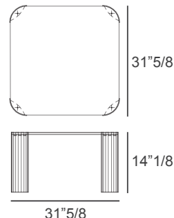
Square - I)
