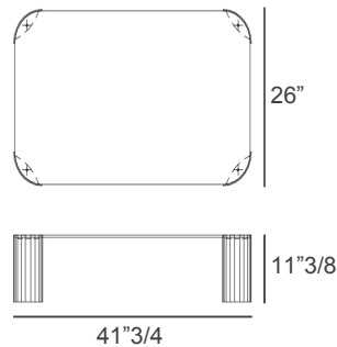
Rectangular - F)
