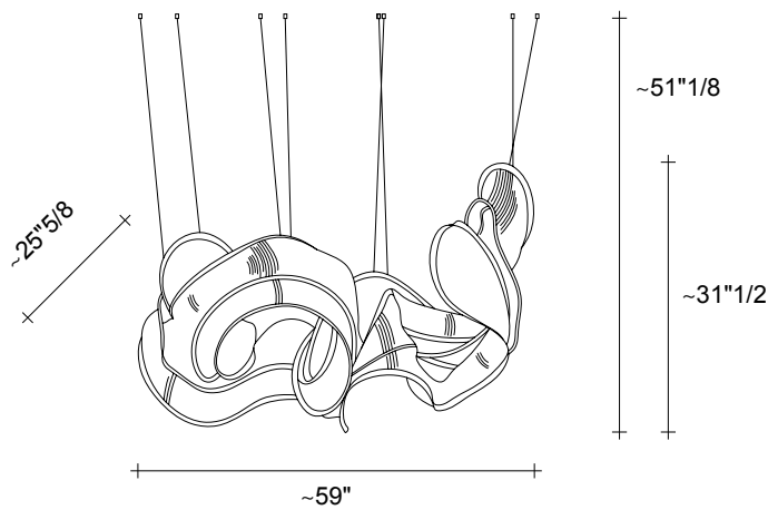
Linear A
