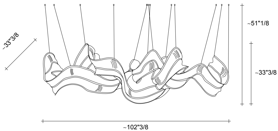
Linear B
