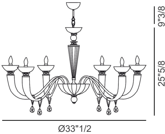
6 ARMS - L6
