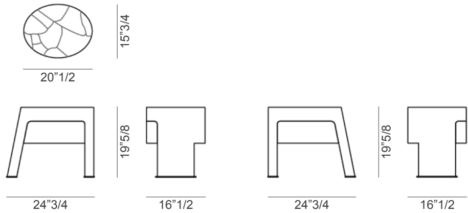
Left side
